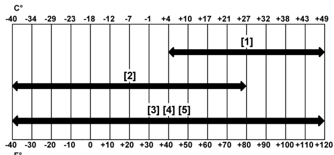
Рис. 255 РЕКОМЕНДУЕМЫЙ КЛАСС ВЯЗКОСТИ ПО ISO (VG) И ИНДЕКС ВЯЗКОСТИ (VI) МАСЛА ГИДРАВЛИЧЕСКОЙ/ГИДРОСТАТИЧЕСКОЙ СИСТЕМЫ
