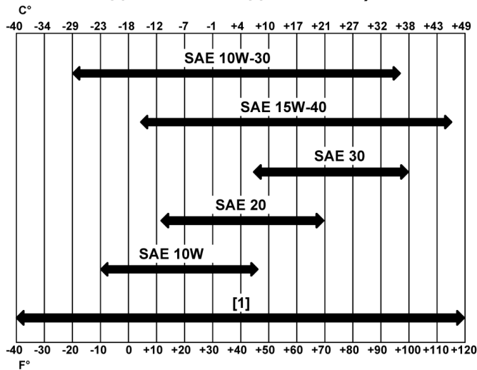
Рис. 227 РЕКОМЕНДУЕМЫЙ КЛАСС ВЯЗКОСТИ ПО SAE МОТОРНОГО МАСЛА (СМАЗОЧНЫЕ МАСЛА ДЛЯ ДИЗЕЛЬНОГО ДВИГАТЕЛЯ)
